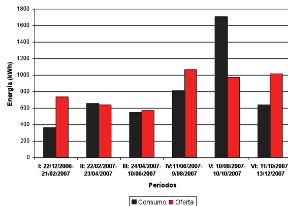
Figura 2. Consumo de energía eléctrica de la escuela de Curiñanco versus la oferta de energía generada, año 2007.
