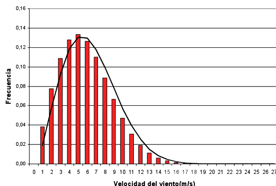
Figura 1. Distribución de frecuencias determinadas a través del modelo estadístico Weibull en el sector de Curiñanco.
